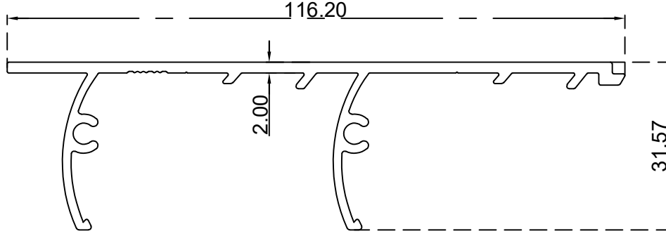
قاعدة رفراف 55 ملم الرقم التسلسلي للصنف: BLT4237 الوزن 1.055:(Kg/m)
