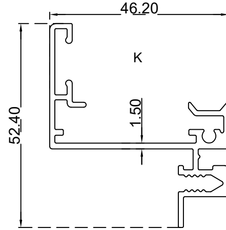
برواز رفراف ثابت الرقم التسلسلي للصنف: BLT1650 الوزن 0.698:(Kg/m)
