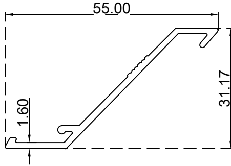
رفراف 55 ملم الرقم التسلسلي للصنف: BLT4238 الوزن 0.336:(Kg/m)
