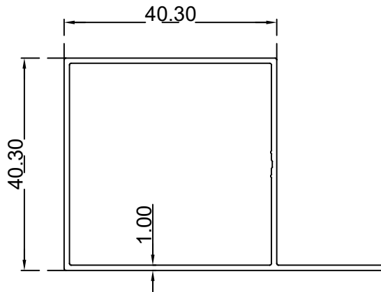
مربع مستور جفيسا الرقم التسلسلي للصنف: AS00066 الوزن 0.482:(Kg/m)
