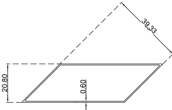
معين خفيف (39.33*20.80) ملم الرقم التسلسلي للصنف: AS00023 الوزن 0.272:(Kg/m)
