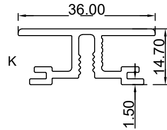
قاعدة رفراف ثابت الرقم التسلسلي للصنف: BLT3943 الوزن 0.446:(Kg/m)
