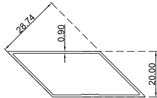
قاعدة رفراف 55 ملم الرقم التسلسلي للصنف: BLT4643 الوزن 1.329:(Kg/m)
