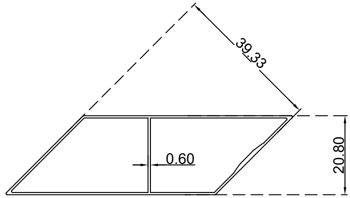
معين خفيف مقوى (39.33*20.80) ملم الرقم التسلسلي للصنف: AS00023B الوزن 0.316:(Kg/m)
