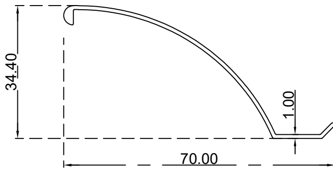
رفراف ثابت 70 ملم الرقم التسلسلي للصنف: BLT1704 الوزن 0.251:(Kg/m)
