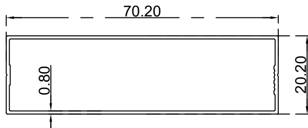
مستطيل (20.20*70.20) ملم الرقم التسلسلي للصنف: BLT3283 الوزن 0.393:(Kg/m)
