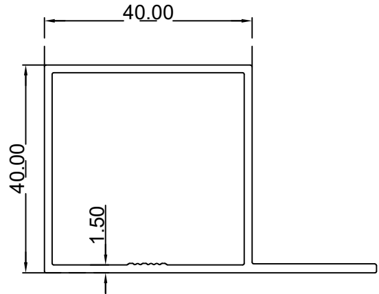
دفة مع كنت (40 /40) ملم الرقم التسلسلي للصنف: BLT3957 الوزن 0.743:(Kg/m)
