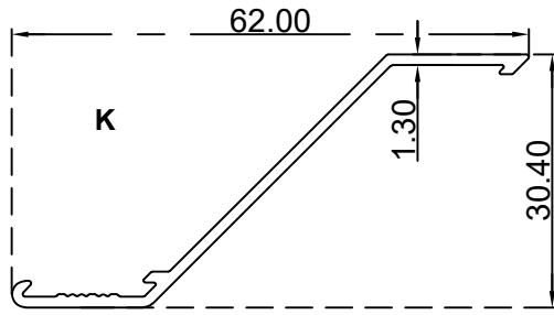
رفراف 55 ملم الرقم التسلسلي للصنف: BLT3793 الوزن 0.284:(Kg/m)
