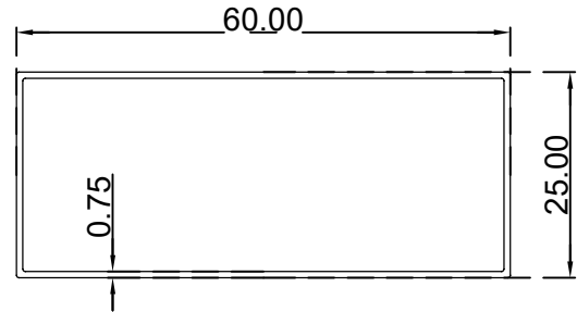
مستطيل (25*60) ملم الرقم التسلسلي للصنف: AS00007B الوزن 0.341:(Kg/m)
