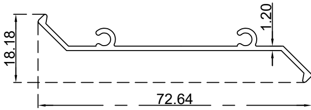
رفراف مع برغرين 72.64 ملم الرقم التسلسلي للصنف: BLT1119 الوزن 0.331:(Kg/m)
